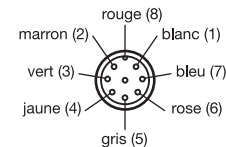
Fiche 8 pôles : positionnement des broches
