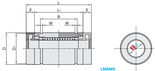
LMBMX 标准型
