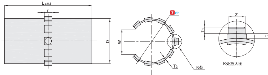
RHDNOP 开口型
