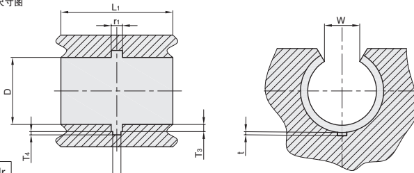
RHDNOP 开口型
