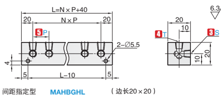
间距指定型 MAHBGHL (边长20×20)
