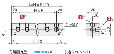
间距固定型 MAHBGJL (边长20×20)
