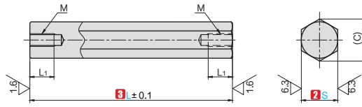
两端内螺纹型
